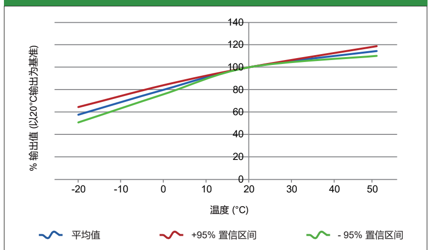
盛密科技民用CO传感器温度性能
