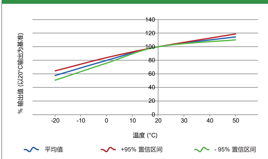
盛密科技民用CO传感器温度性能
